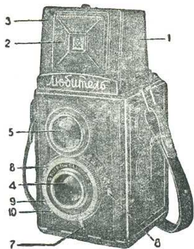
1—светозащитные шторки; 2—щиток с заводской маркой; 3—передняя рамка; 4—фотообъектив; 5—объектив видоискателя; 6—рычаг регулировки диафрагмы; 7—поводок регулировочного кольца затвора; 8—заводной рычаг затвора; 9—спусковой рычаг затвора; 10—резьбовое гнездо для тростика
