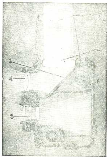
1—установочная лупа; 2—коллективная линза видоискателя с матовым кружком внизу; 3—зеркало; 4—объектив видоискателя; 5—фотообъектив; 6—фотопленка
